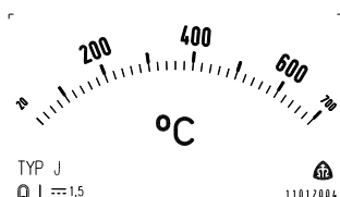
[4] Stupnice pro teploměry
