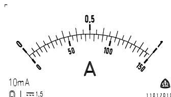
[6] Stupnice pro ampérmetr se dvěma rozsahy
