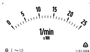
[5] Stupnice pro otáčkoměry
