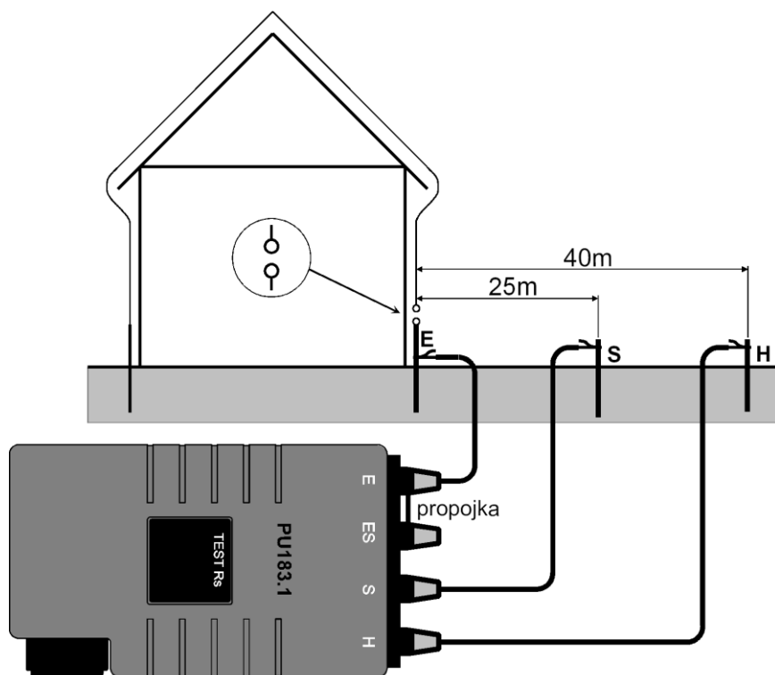
obr.5 třívodičové připojení
