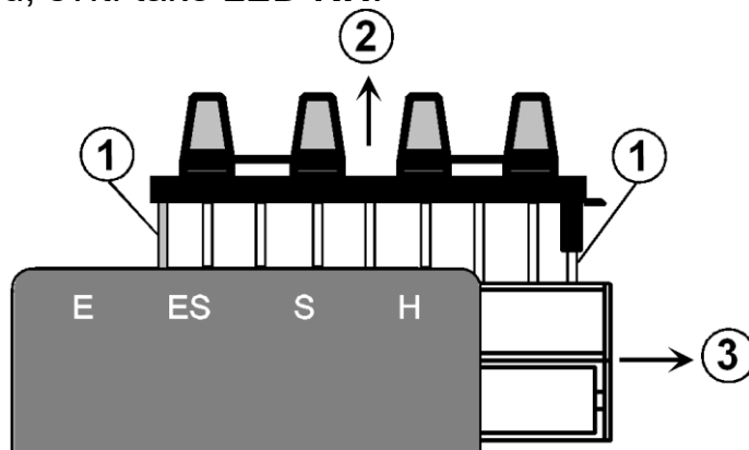
Obr.4 vkládání akumulátorů
