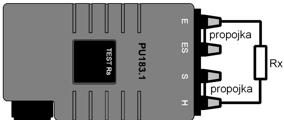
obr.7 měření ohmického odporu
