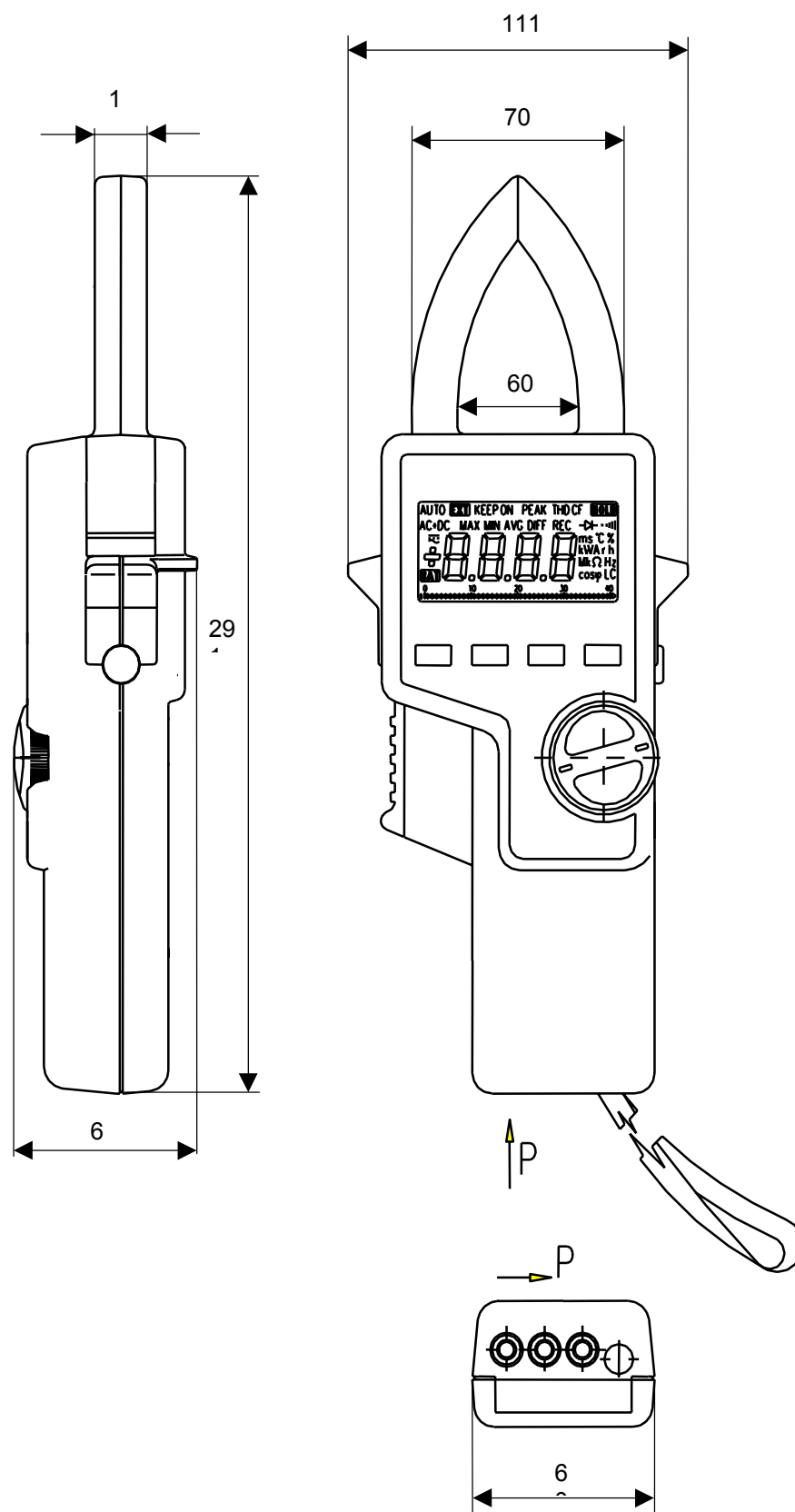
Obr.1. Rozměrový náčrtek
